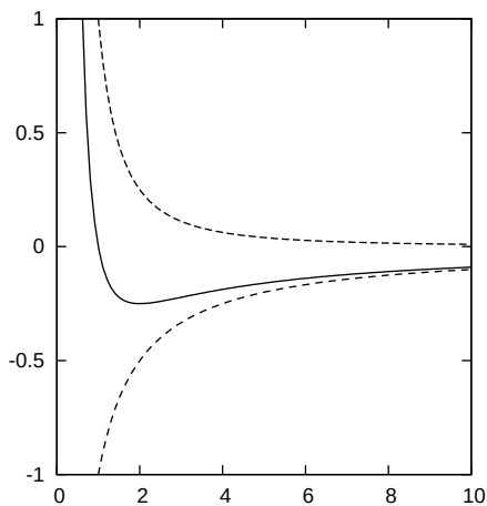
図 2.3 万有引力における有効ポテンシャル。
