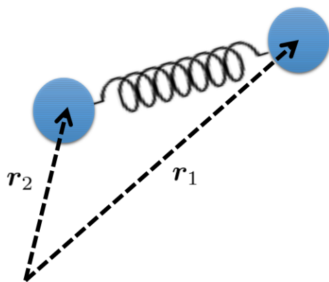
図 2.5 2次元中の2粒子に対するバネの運動。
