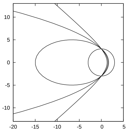
図 2.4 万有引力のニュートン方程式を解くことで得られる軌道。
